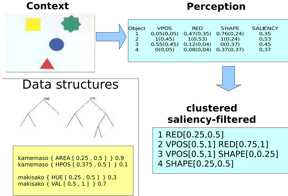
FIG. 2.4 – Déroulement de la perception des agents et structures de données
